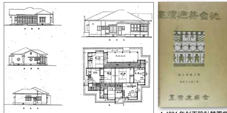
▲1930年住宅設計競圖第一等當選圖案。（圖片來源：《臺灣建築會誌》第二輯第三號）。
